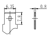
terminal F2(optional)
